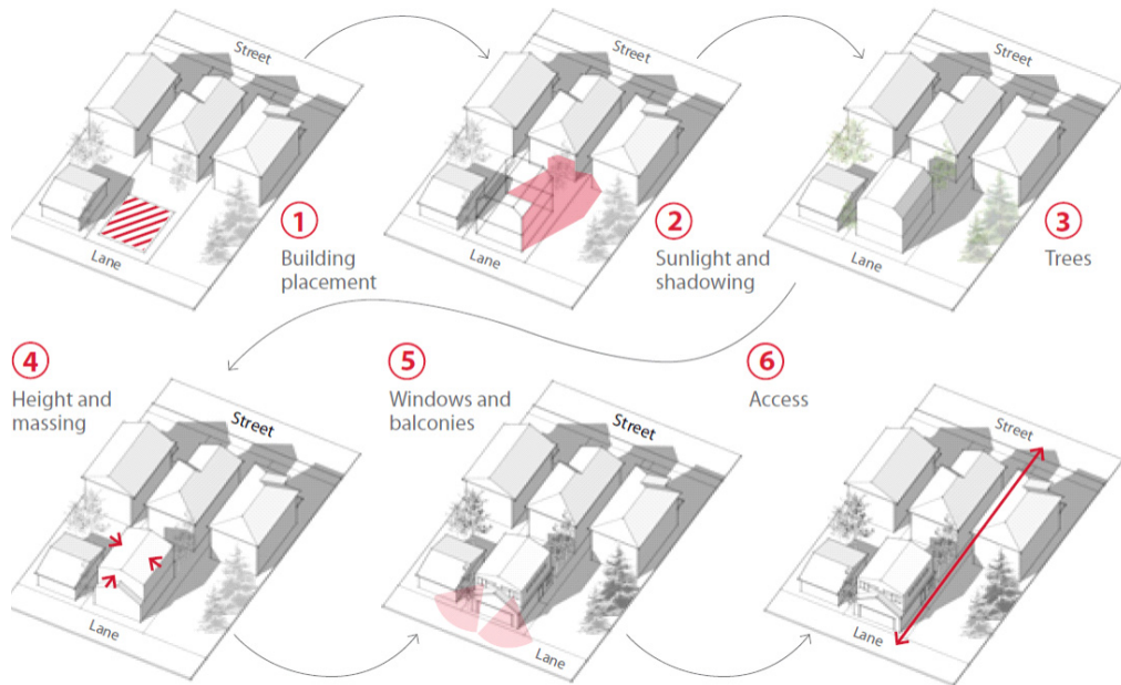
[그림] 뒷마당 추가 주택 설계 시 고려해야 할 6가지 요소를 보여주는 입체도
